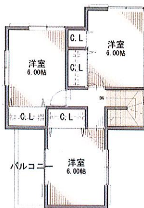
2階平面図
