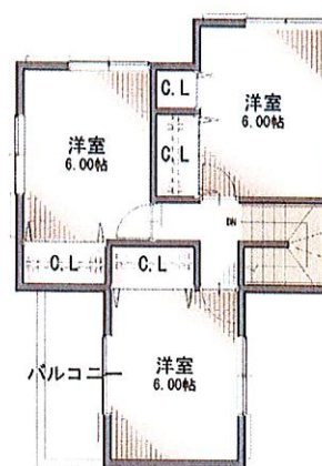
2階平面図
