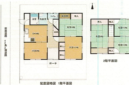
配置図略図 1階平面図
