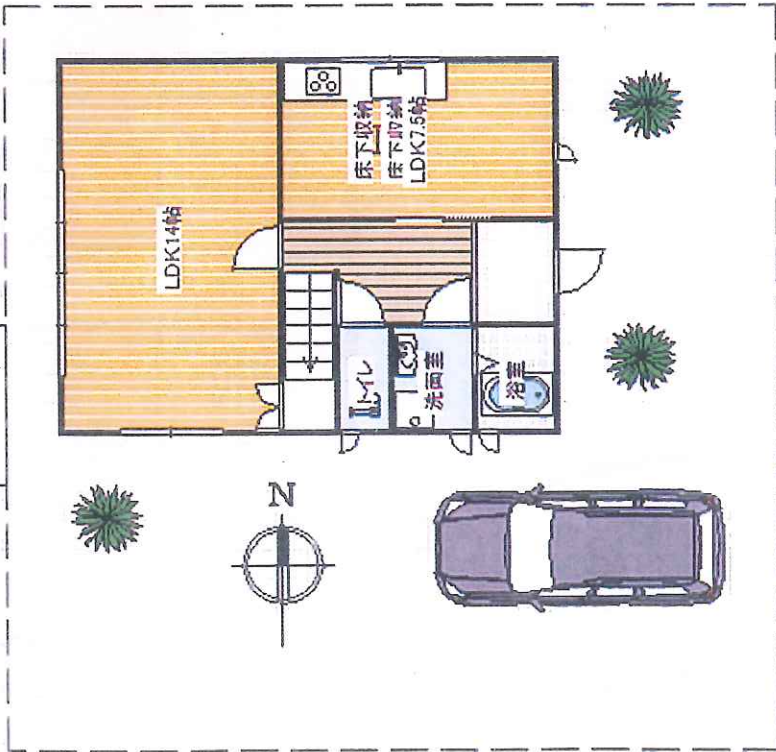
1階平面図
