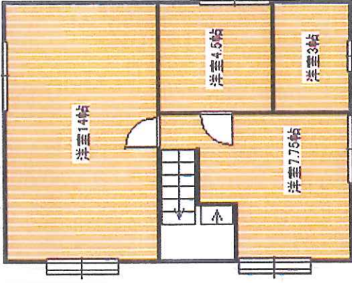
2階平面図
